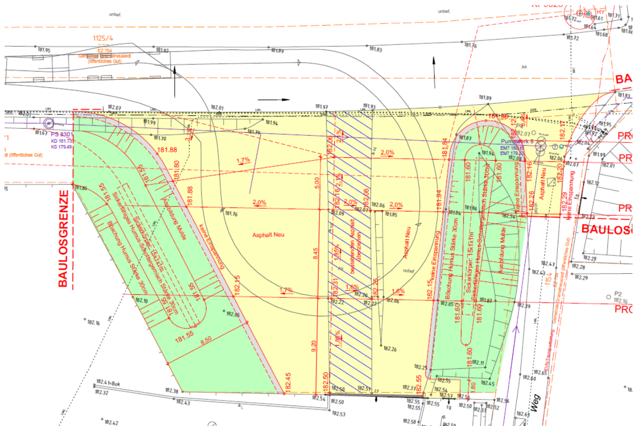
Abbildung 4 Ausschnitt aus Projektplan DI Paikl PlanNr. 1568/10 v. April 2023
